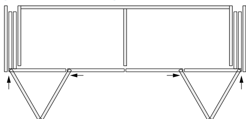
Hawa Folding Concepta III 25 Push, izquierda/derecha Aluminio, anodizado
